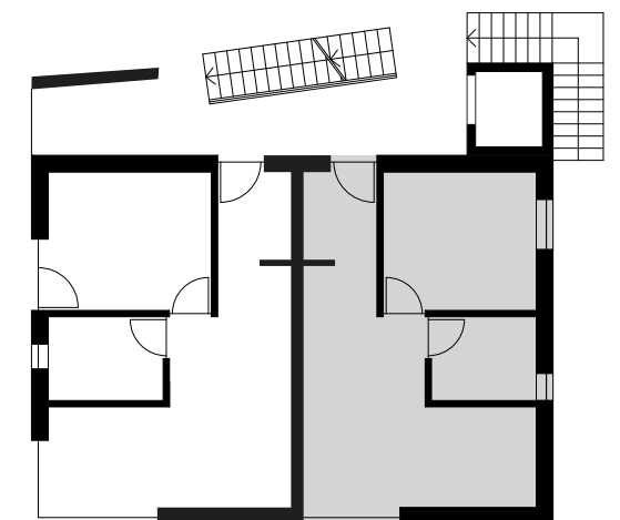
Erdgeschoss Übersichtsplan
