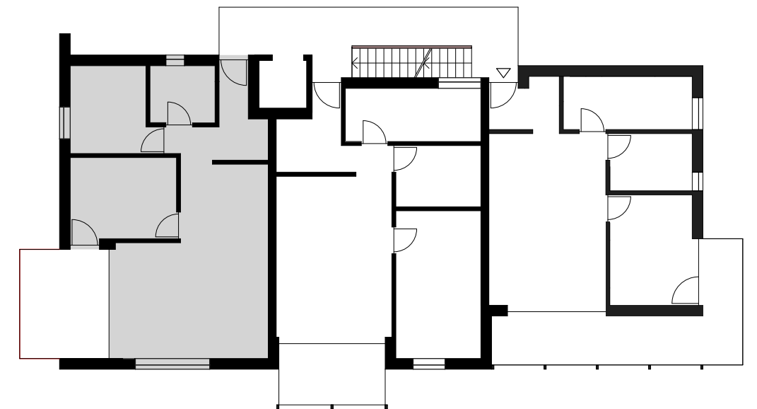
2. Obergeschoss Übersichtsplan
