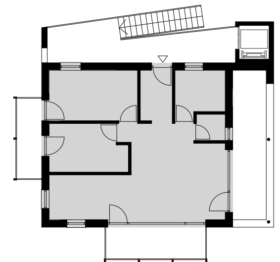
2.Obergeschoss Übersichtsplan
