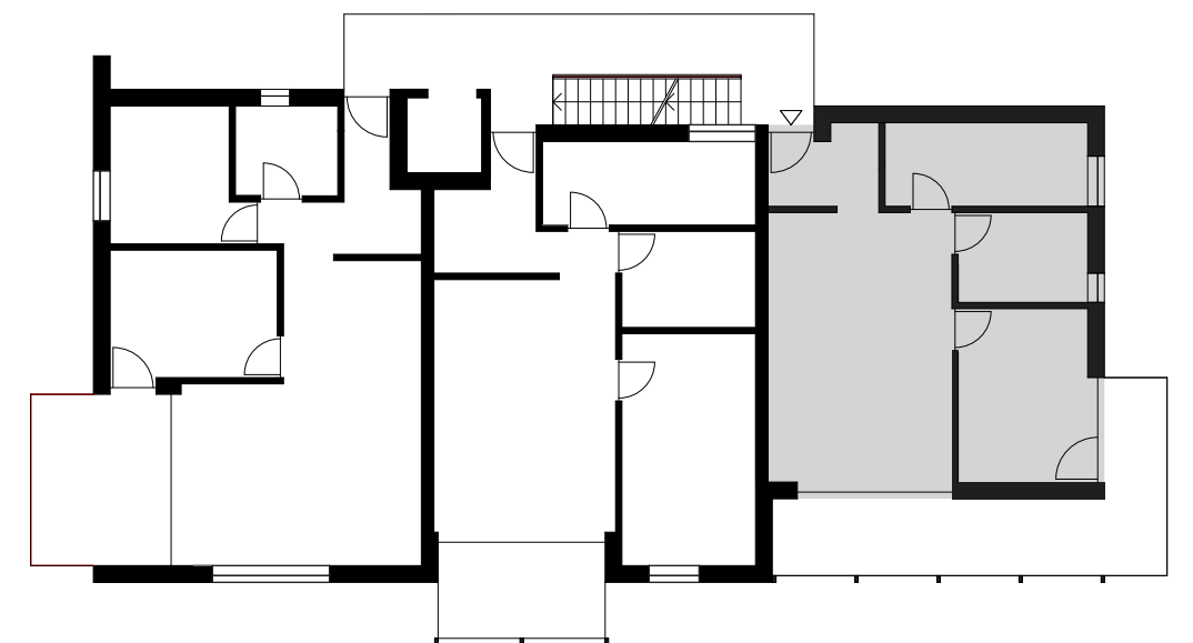
1. Obergeschoss Übersichtsplan
