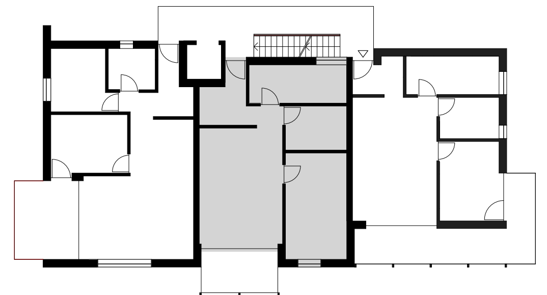
2. Obergeschoss Übersichtsplan
